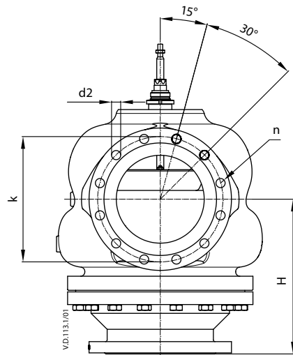
VF 3 (DN 250-300)
